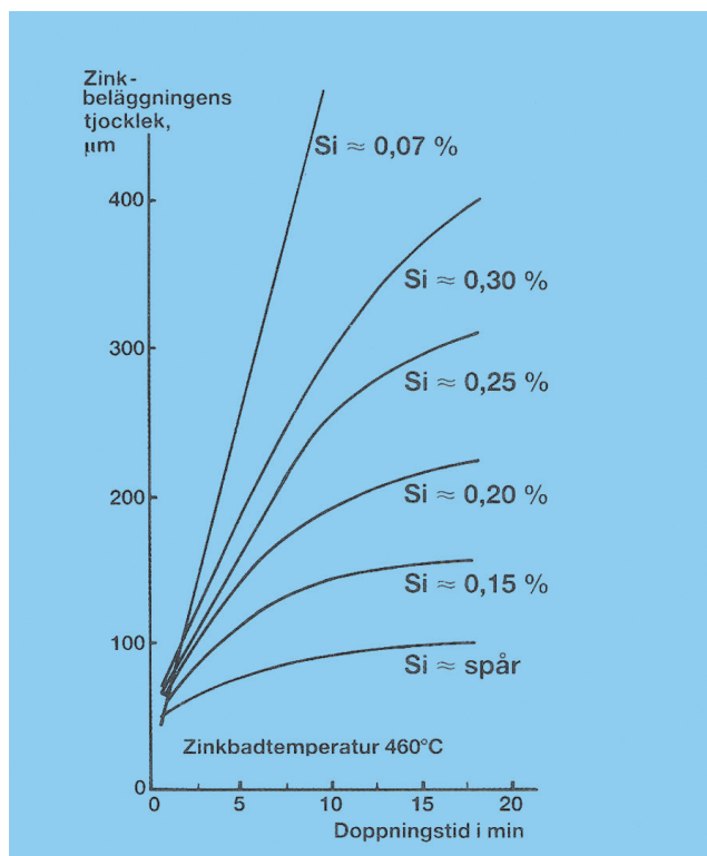
Figur 1. Relationen mellan dopningstid och zinkskiktets tjocklek för stål med olika kiselhalter. Kurvorna är medelkurvor baserade på såväl undersökningar som praktiska erfarenheter. Betydande variationer kan förekomma mellan stål med lika kiselhalter men från olika charger.
