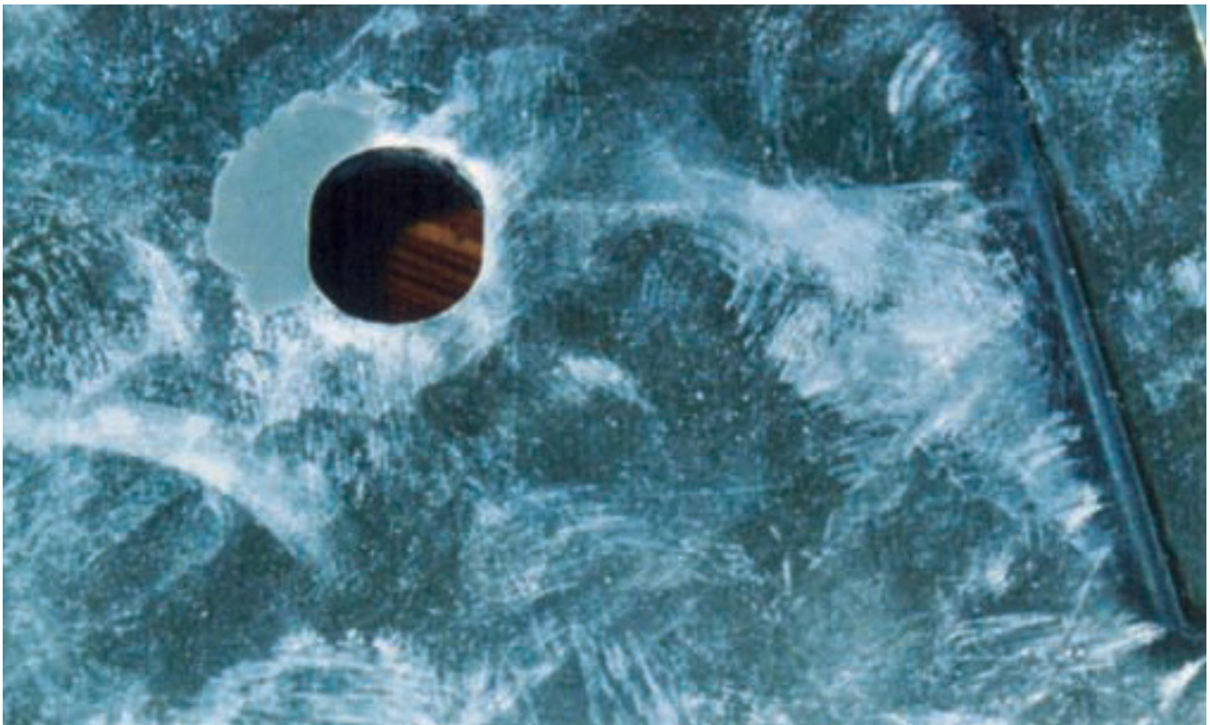
Eksempel på reparation af zinkafskalning omkring et udstanset hul i varmforzinket plade. Reparationen er udført med zinkmaling.
